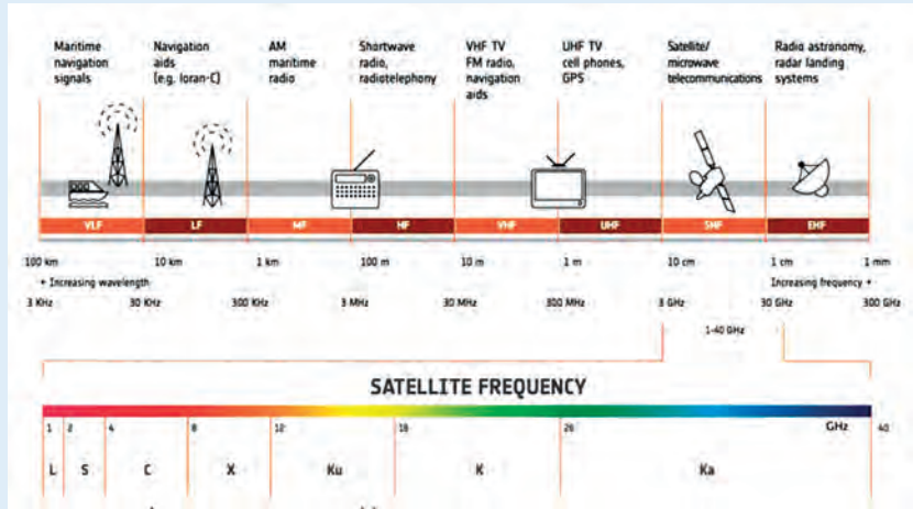
ภาพที่ ๗ แผนภาพแสดงย่านความถี่ที่ถูกนำมาใช้งานสำหรับกิจการอวกาศ โดยการใช้ตัวอักษรกำกับ
