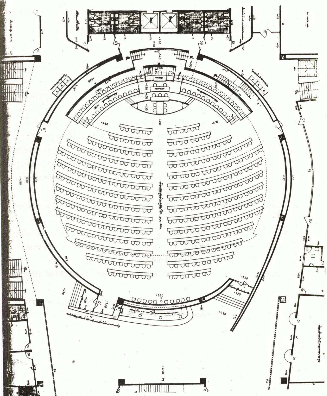
ผังแสดง ห้องประชุมสภา ที่นั่งสมาชิกสภา ๔๐๐ ที่
