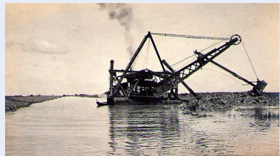
การใช้เครื่องจักรขุดคลอง
