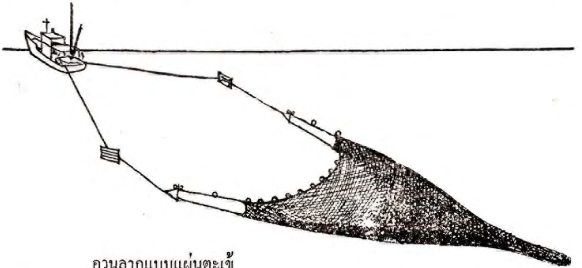
อวนลากมีคานถ่าง
