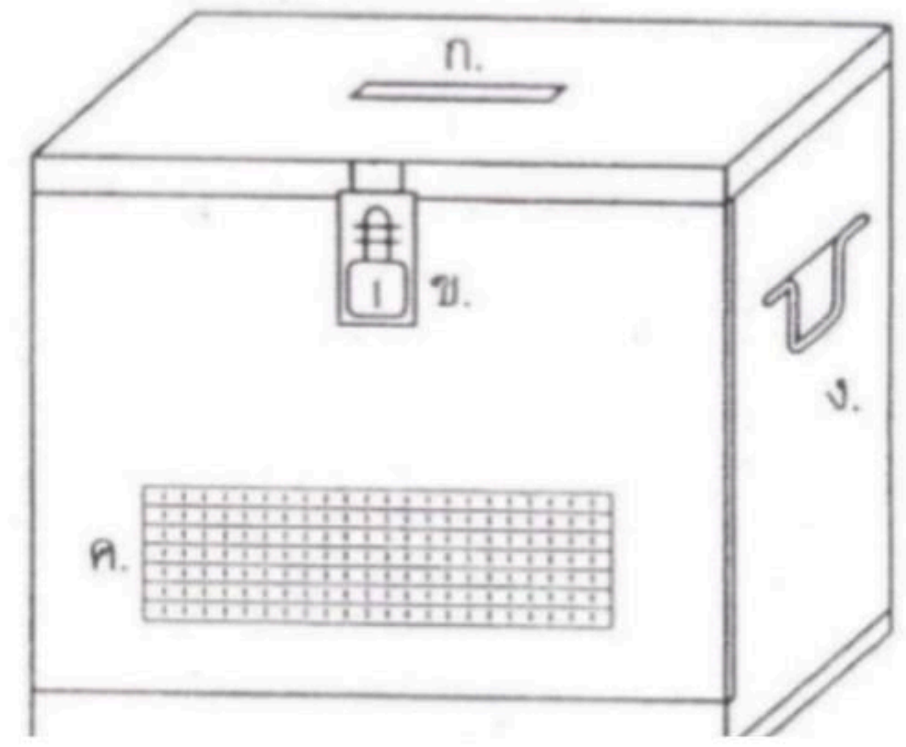
2 แบบที่ 2 ก. - ช่องใส่บัตรเลือกตั้ง ข. - กุญแจหรืออุปกรณ์อื่นแทนกุญแจ ค. - วัสดุที่สามารถมองเห็นภายในหีบฯ ง. - หูสำหรับยกหีบฯ
