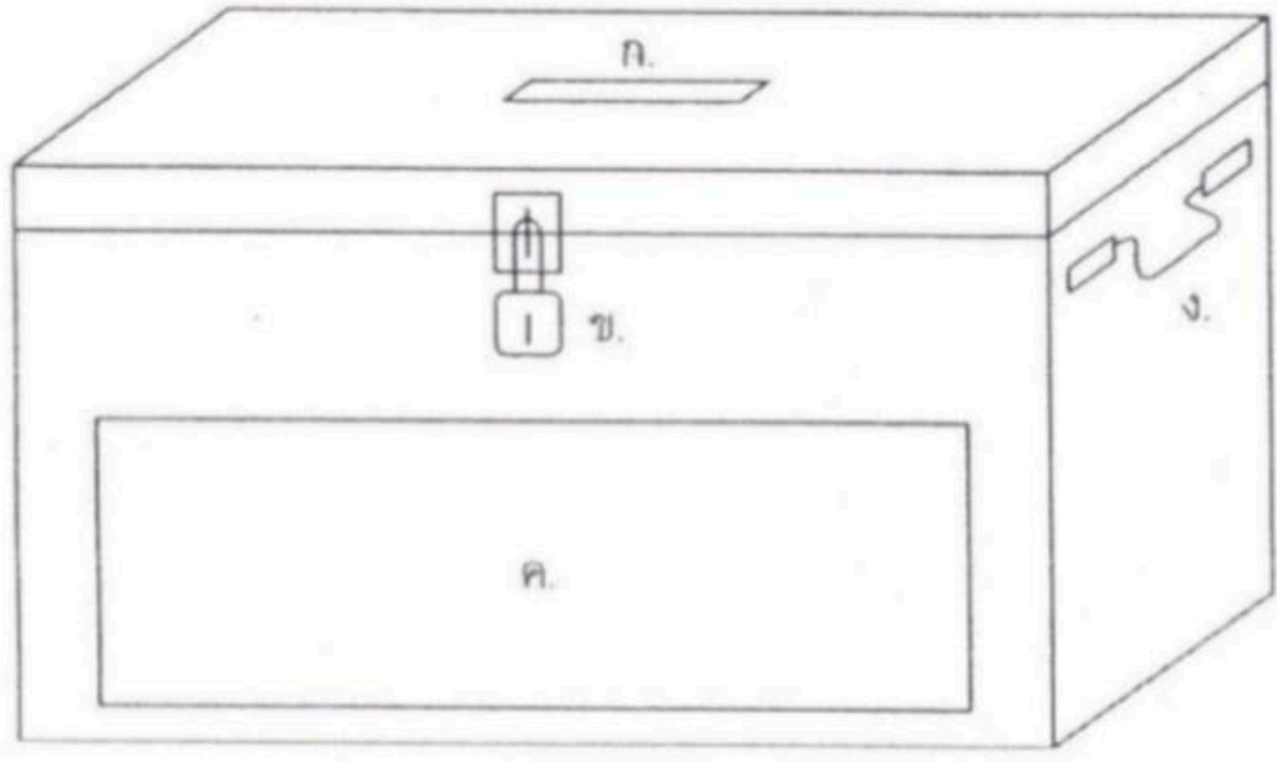
1 แบบที่ 1 ก. - ช่องใส่บัตรเลือกตั้ง ข. - กุญแจหรืออุปกรณ์อื่นแทนกุญแจ ค. - วัสดุที่สามารถมองเห็นภายในหีบฯ ง. - หูสำหรับยกหีบฯ
