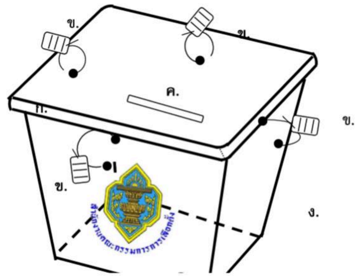
4 แบบที่ 4 ก. - ฝาปิดหีบฯ ข. - สายรัด 4 เส้น ค. - ช่องใส่บัตรเลือกตั้ง ง. - วัสดุที่สามารถมองเห็นภายในหีบฯ จ. ตราสัญลักษณ์ สنج. คณะกรรมการการเลือกตั้ง
