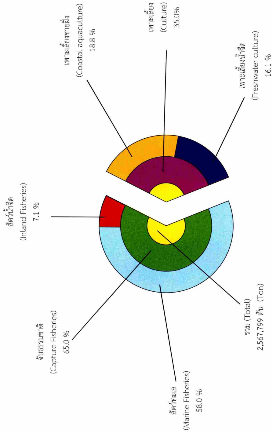
แผนภูมิที่ 3 ปริมาณการจับสัตว์น้ำทั้งหมด จำแนกตามวิธีการทำประมง ปี 2557 Chart No. 3 Fisheries production in quantity by sub-sector, 2014
