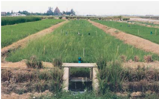
ภาพที่ 1 ลักษณะสังเขปรูปแบบเทคโนโลยีการบำบัดน้ำเสียด้วยระบบหน้ากรบน้ำเสีย
