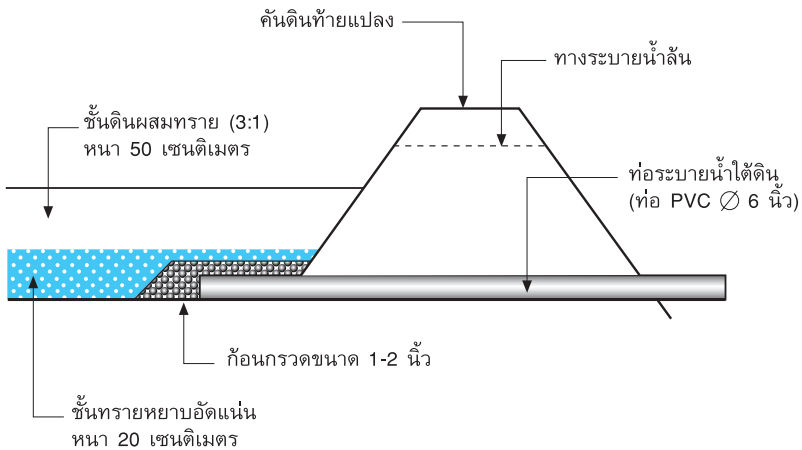
ภาพที่ 6 ลักษณะการวางท่อระบายน้ำใต้ดินท้ายแปลงระบบพญากรองน้ำเสีย
