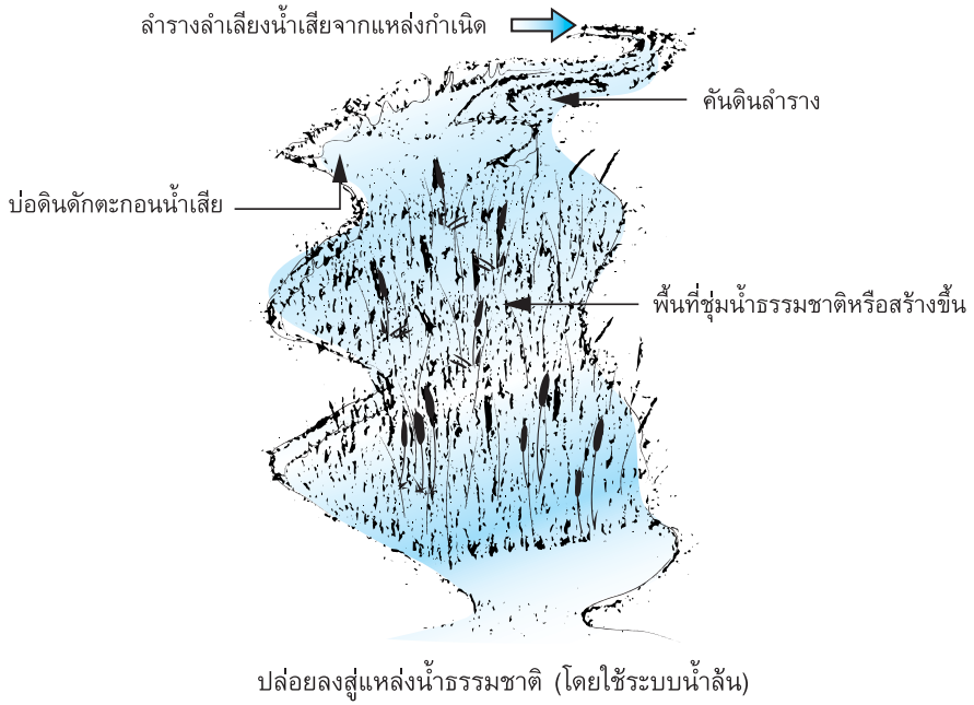
ภาพที่ 9 แนวคิดในการปรับปรุงพื้นที่ใช้เป็นระบบบำบัดน้ำเสียด้วยพื้นที่ชุ่มน้ำเทียม
