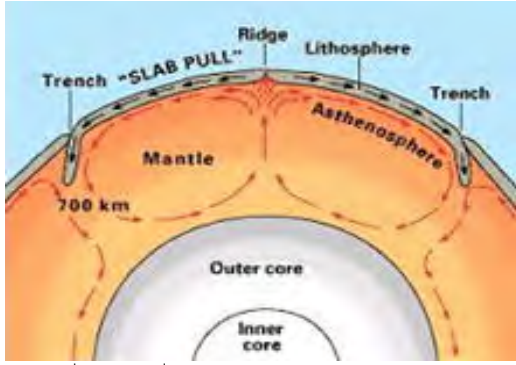
รูปที่ 1 การเคลื่อนตัวของหินหลอมละลายภายในโลก
