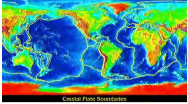
รูปที่ 2 แนวแผ่นดินไหวของโลก
