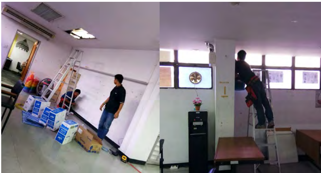
การติดตั้งจุดเชื่อมต่อเครือข่ายคอมพิวเตอร์ ปลั๊กไฟ และจุดเชื่อมต่อสายโทรศัพท์
