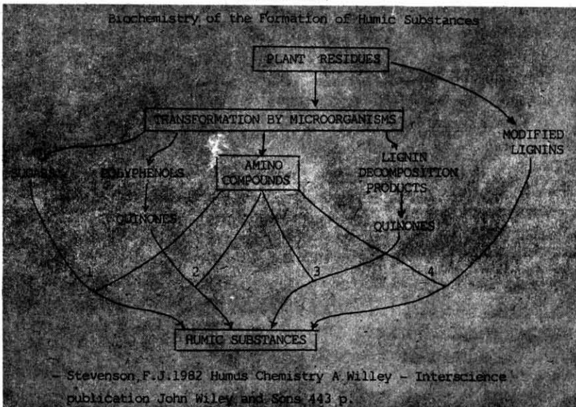
รูปที่ 1 ขบวนการกำเนิด ฮิวมิก แอซิด (humic substances)
