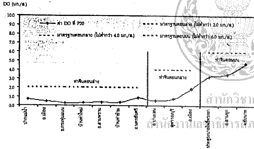
รูปที่ 2 ค่าเปอร์เซ็นต์ไอล์ที่ 20 ของปริมาณออกซิเจนละลาย (DO) ในแม่น้ำท่าจีน จำแนกตามสถานีตรวจวัด ตั้งแต่ปี 2538-2547
