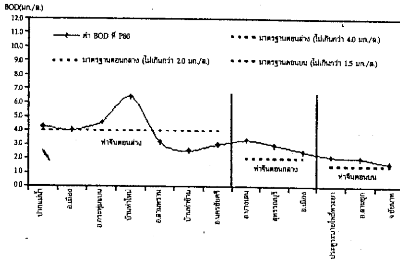
รูปที่ 3 ค่าเปอร์เซ็นต์ไอล์ที่ 80 ของปริมาณความสกปรกในรูปสารอินทรีย์ (BOD) ในแม่น้ำท่าจีน จำแนกตามสถานีตรวจวัด ตั้งแต่ปี 2538-2547
