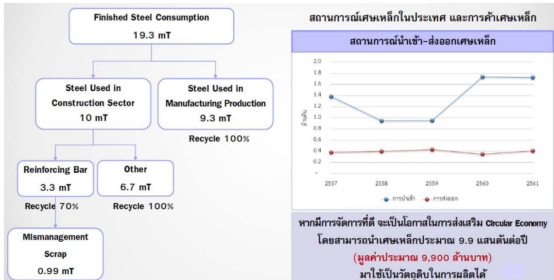
แผนภาพที่ ๔ - ๒ ภาพรวมสถานการณ์เศษเหล็กและปริมาณการหมุนเวียน
